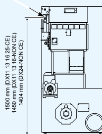
Arrière DX 11 13 16 24 Gaz
