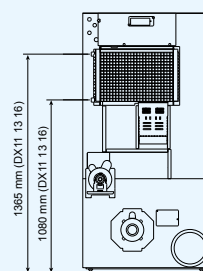
Arrière DX 11 13 16 Vapeur
