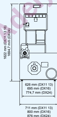
Arrière DX 11 13 16 24 Electrique
